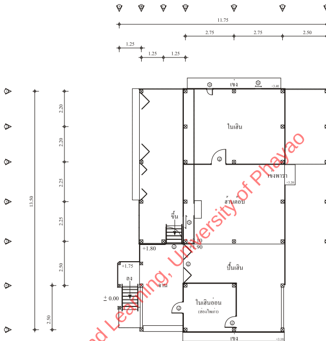
ภาพวาดลายเส้นผังเรือนพักอาศัยของคุณคำหลู่ สุนันท์ บ้านเมืองปอน
